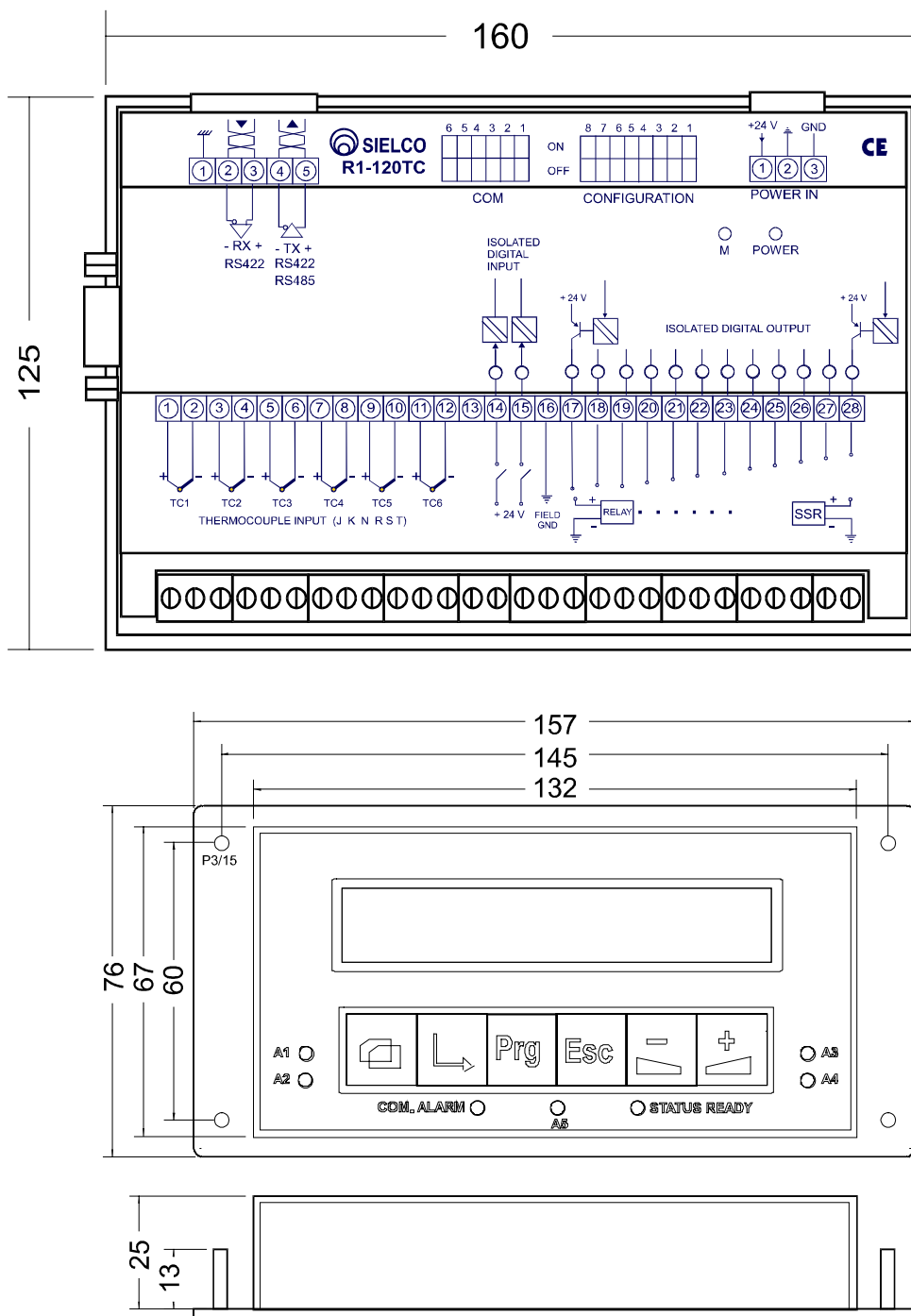
Figura 1.1 - Dimensioni del modulo D1-60AV e del pannello operatore F1-10
