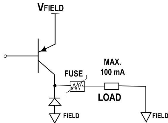
Figura 1.4 - Uscite logiche.
