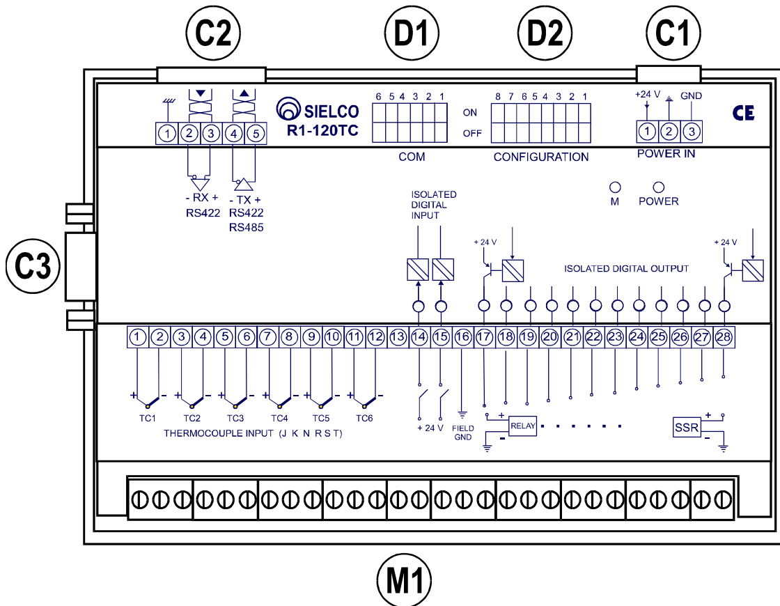
Figura 1.3 - Schema R1-120TC e F1-10.
