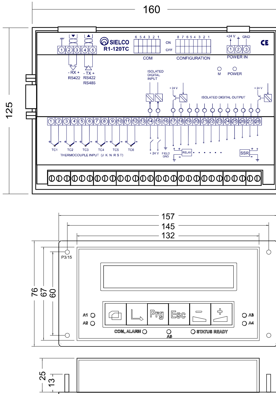
Figura 1.1 - Dimensioni del regolatore R1-120TC.
